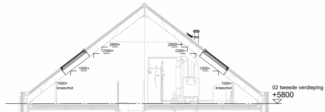
Doorsnede schaal 1:100
