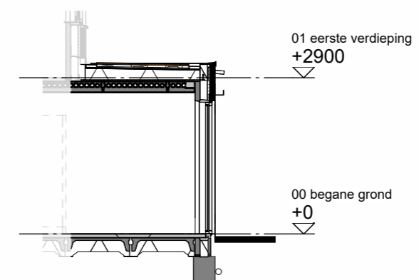
Doorsnede schaal 1:100
