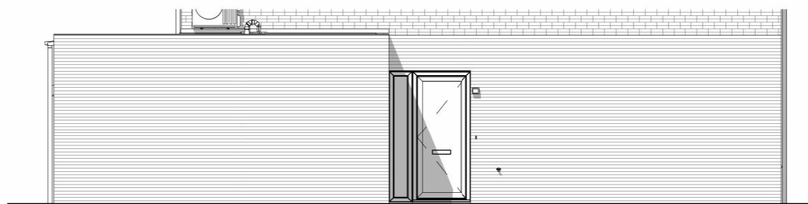
Linkerzijgevel schaal 1:100
