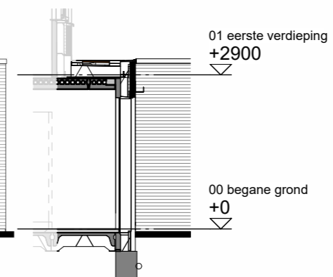
Doorsnede schaal 1:100
