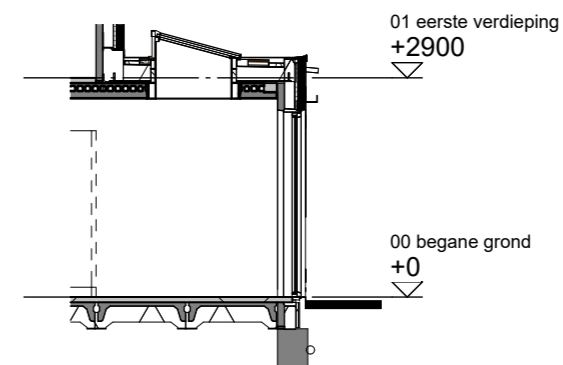
Doorsnede schaal 1:100
