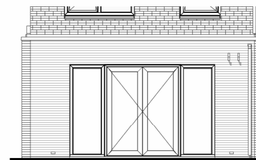
Achtergevel schaal 1:100
