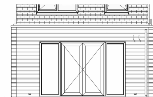
Achtergevel schaal 1:100
