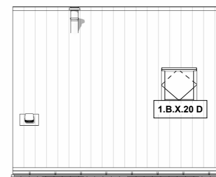
Voorgevel schaal 1:100
