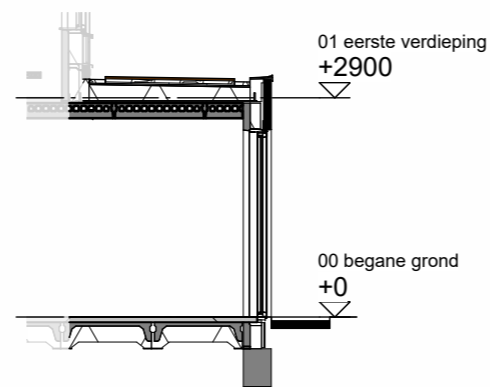
Doorsnede schaal 1:100
