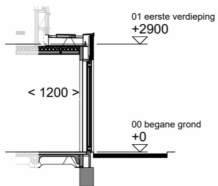
Doorsnede schaal 1:100
