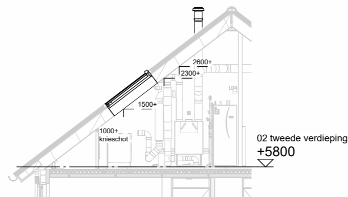
Doorsnede schaal 1:100
