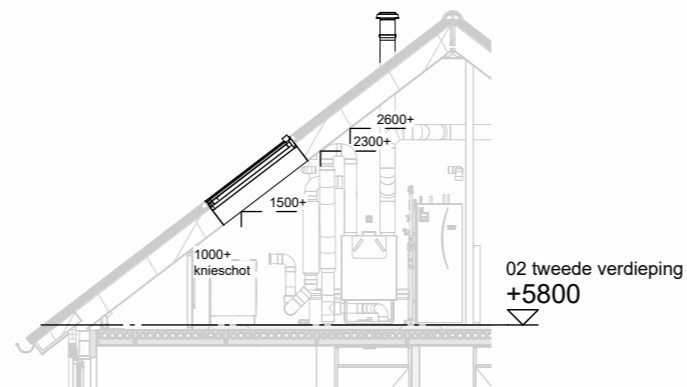
Doorsnede schaal 1:100
