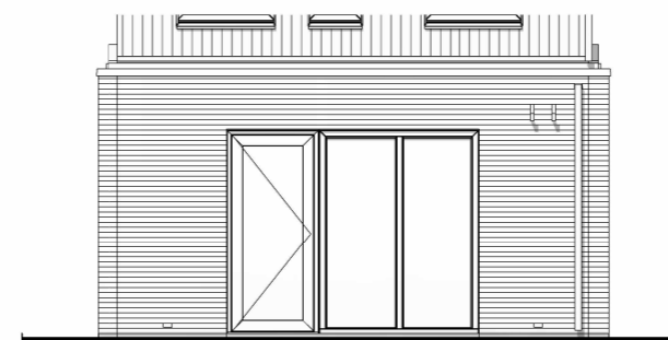
Achtergevel schaal 1:100
