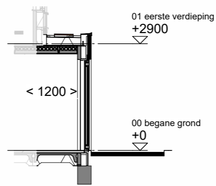
Doorsnede schaal 1:100
