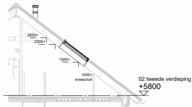
Doorsnede schaal 1:100
