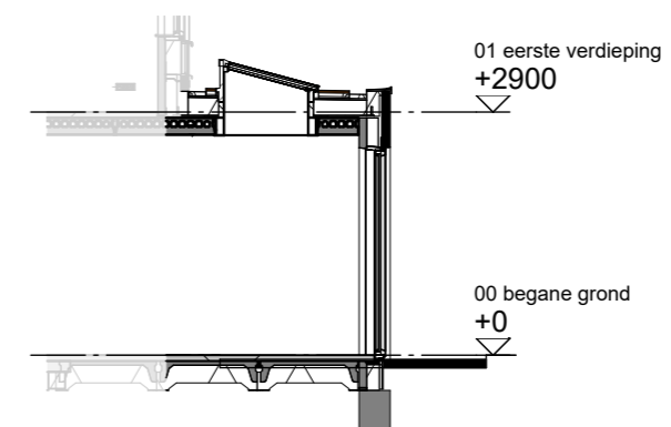
Doorsnede schaal 1:100
