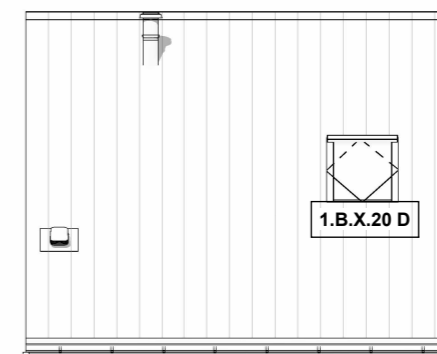
Voorgevel schaal 1:100
