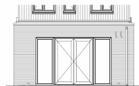
Achtergevel schaal 1:100
